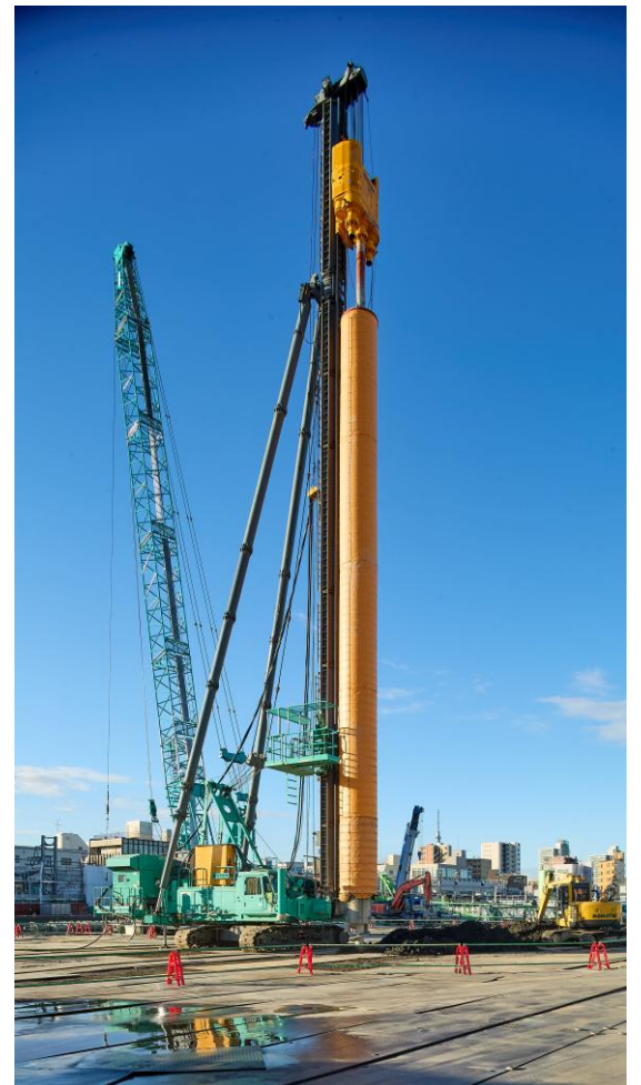
山留工事（東街区）
